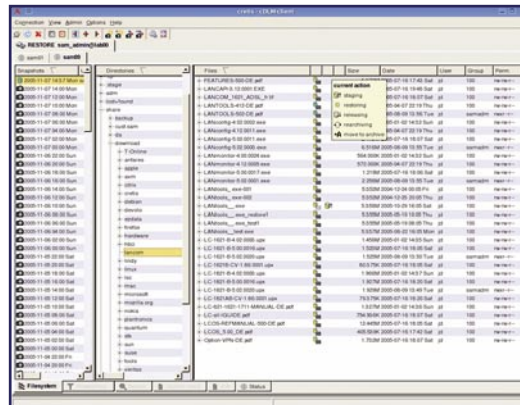
Linux
