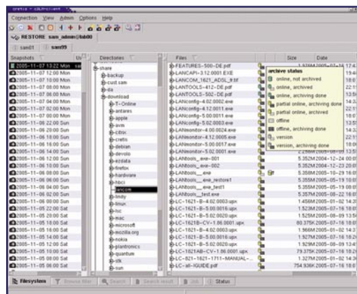
Solaris
